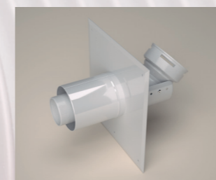
přípojovací deska DN60/100-80
