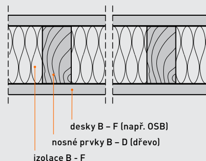
Konstrukční část druhu DP3
