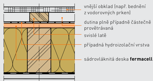
Účinná ochrana proti povětrnostním vlivům provětrávanou fasádou a) případně b).
