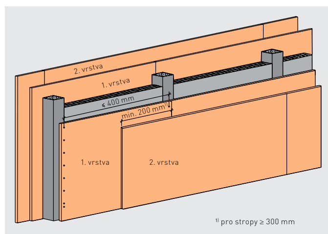
Upevnění desky na desku
