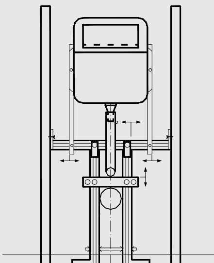
Nosný rám pro závěsné WC se zabudovanou splachovací nádrží.
