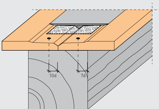
Vzdálenosti od okraje pro TB hrany
