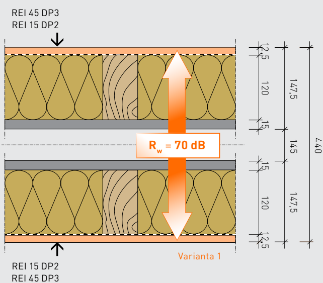
Varianta 1 – Zmenšení mezery mezi vrstvami ze 145 mm na 35 mm → snížení ca -2dB
