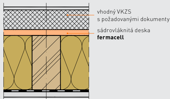
Účinná ochrana proti povětrnostním vlivům prostřednictvím VKZS.
