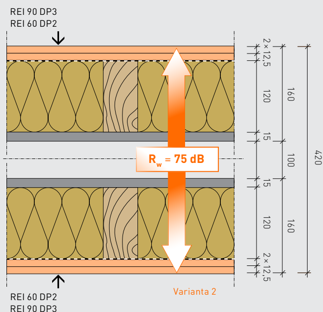
Varianta 2 – Jednovrstvé opláštění na straně místnosti → snížení ca -7dB
