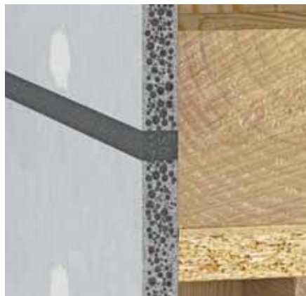
Obr. 4: Uzavření spáry předkomprimovaným těsnícím pásem (detail)
