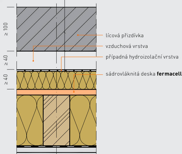
Účinná ochrana proti povětrnostním vlivům lícovou přizdívkou.
