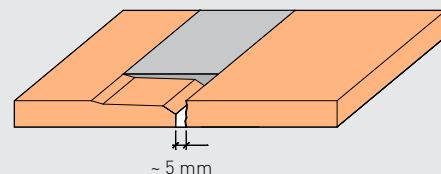
Varianta spáry 3: Jedna TB hrana z výroby a jedna hrana odříznutá na stavbě se spárovacím tmelem fermacell
