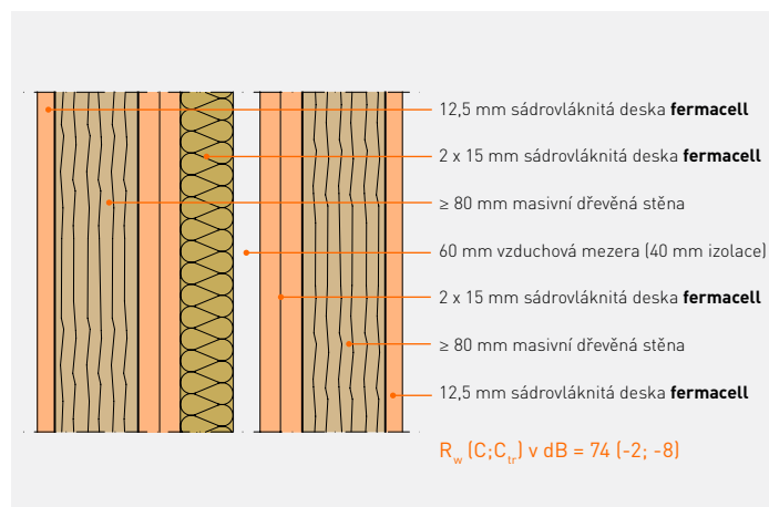
Dělicí stěna mezi domy – opatření pro nízké kmitočty (příklad)
