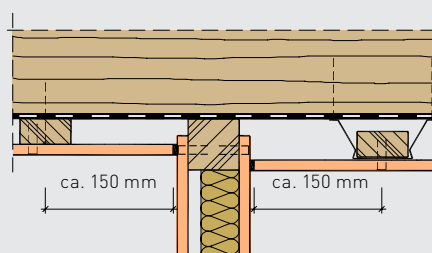
Napojení stropu na stěnu
