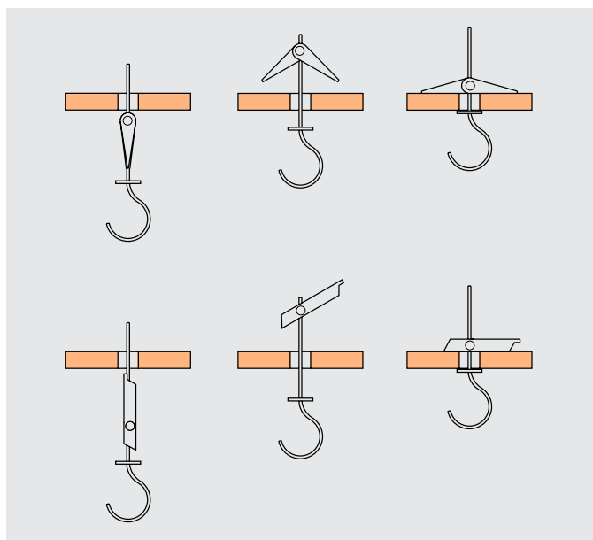
Hmoždinky pro namáhání osovým tahem (rozpěrná a sklopná hmoždinka)
