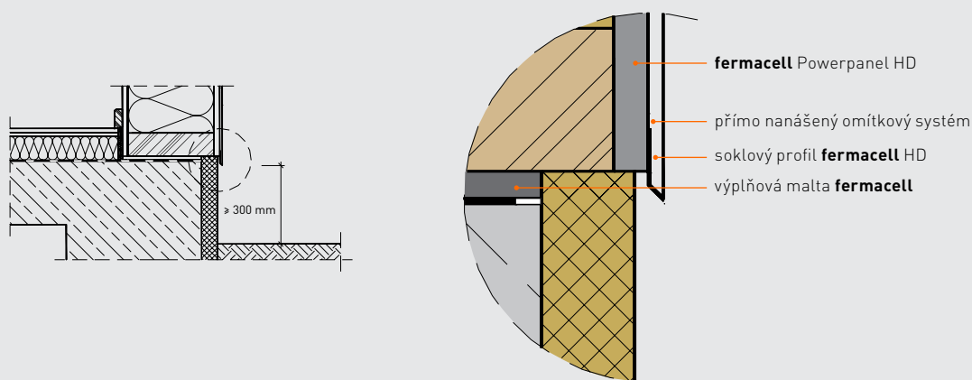
Obr. 1: Připevnění desky Powerpanel HD v oblasti soklu
