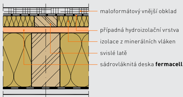
Účinná ochrana proti povětrnostním vlivům bez provětrání.
