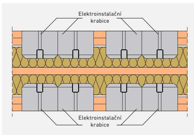
Příklad řešení s přepážkou tvořenou pásy desek a izolací z minerálních vláken mezi elektroinstalačními krabicemi
