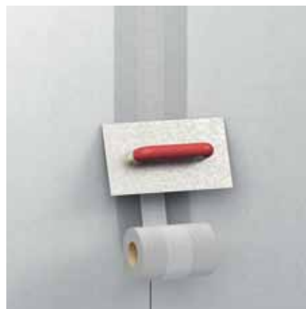
Nanášení armovacího pásky fermacell HD
