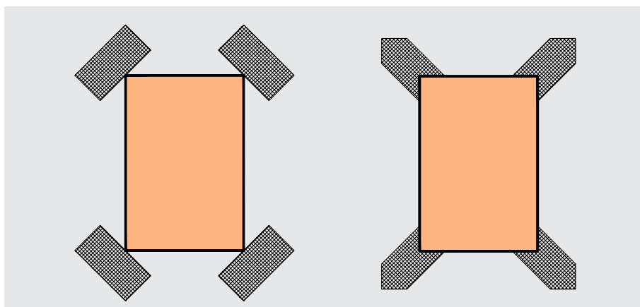
Diagonální armování na okenních a dveřních otvorech pomocí proužků z prořezů (30 x 60 cm armovací tkaniny fermacell HD), popř. „šipek z tkaniny.“
