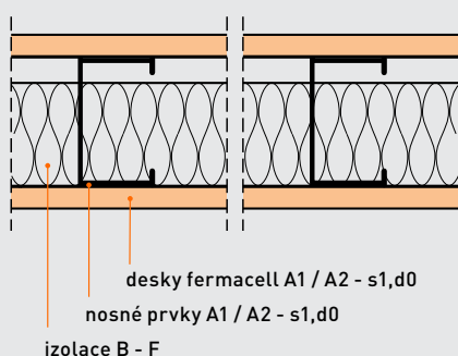
Konstrukční část druhu DP1
