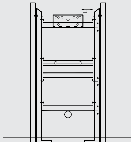
Nosný rám pro umyvadlo, pisoár nebo výlevku
