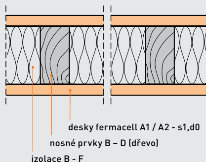
Konstrukční část druhu DP2
