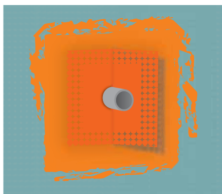
Utěsnění prostupů potrubí se provede pomocí těsnící manžety, která se vtlačí do ještě vlhké tekuté fólie fermacell a ihned se tekutou fólií přetře
