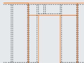
Dveřní otvor při vodorovném styku opláštění
