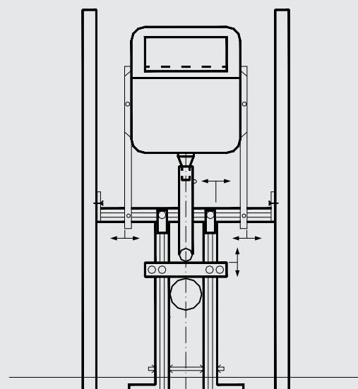
Nosný rám pro závěsné WC s vestavěnou splachovací nádrží
