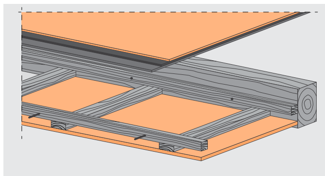
Upevnění se spodní dřevěnou konstrukcí
