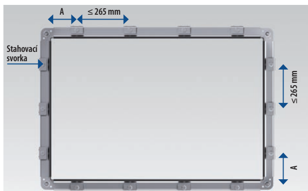
Obr. 61 Rozmístění stahovacích svorek
