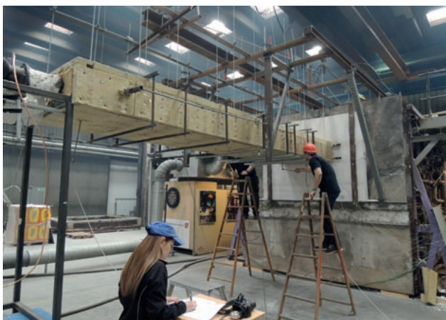
Obr. 72 Měření deformace potrubí typu C při zkoušce ve zkušební
