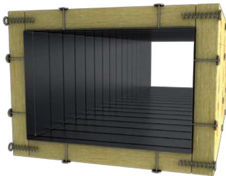
Obr. 63 Horní deska překrývá boční desky, které překrývají spodní desku
