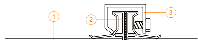
Obr. 11 Rozmístění stahovacích svorek 1 - VZT potrubí 2 - keramická páska 20 × 3 mm 3 - stahovací svorka se šroubem M8 4 - šroub M10 s matkou a podložkou
