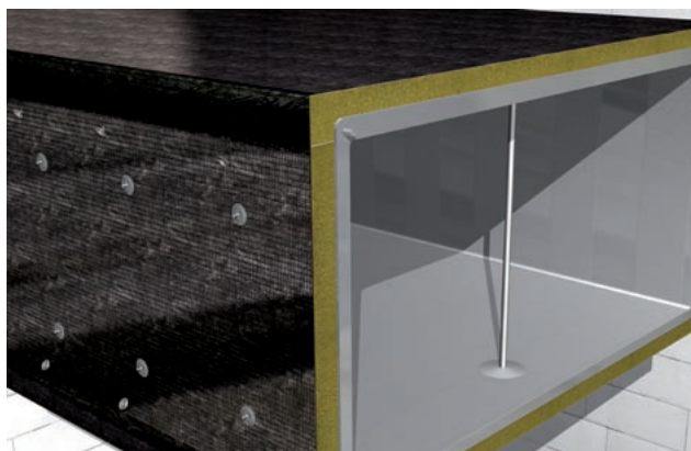
Obr. 32 Vyztužení segmentu potrubí uprostřed rozpětí
