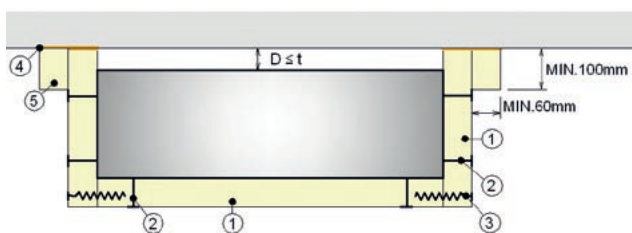
Obr. 46 Příčný řez vodorovným vzduchovodem s izolací na 3 stranách
