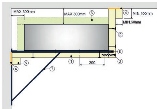
Obr. 47 Příčný řez vzduchovodem s dvoustrannou izolací v místě požárně dělicí konstrukce
