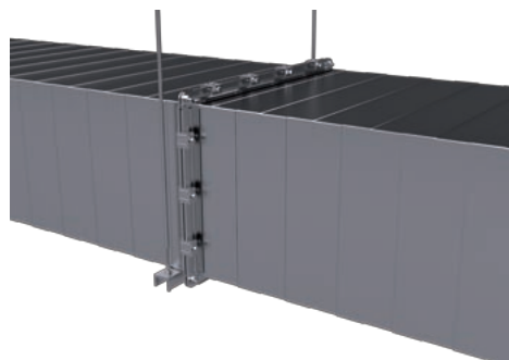
Obr. 62 Závěsné zařízení je možno s výhodou umísťovat do těsné blízkosti přírub
