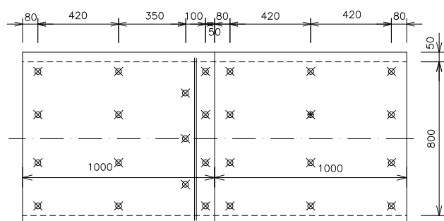
Obr. 30 Příklad rozmístění trnů u kruhového VZT potrubí
