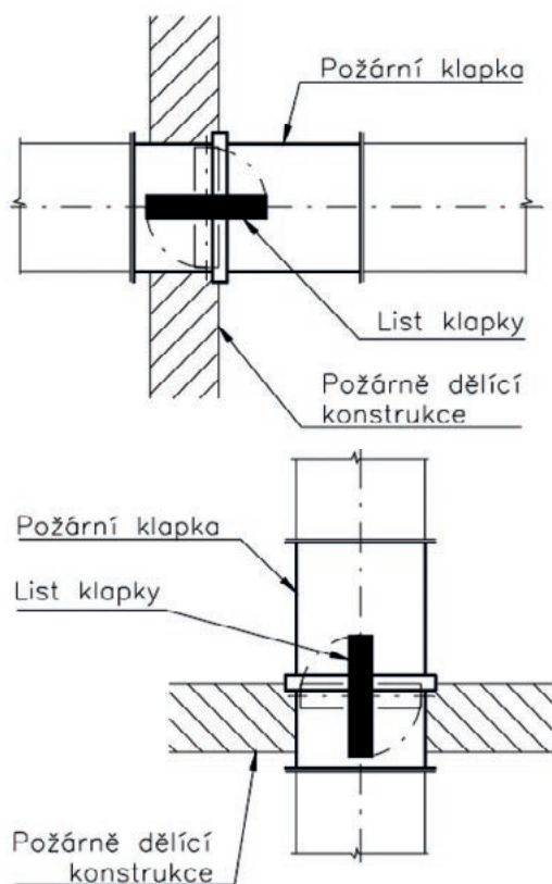
Obr. 80 Požární klapka zabudovaná přímo v požárně dělicí konstrukci svislé nebo vodorovně
