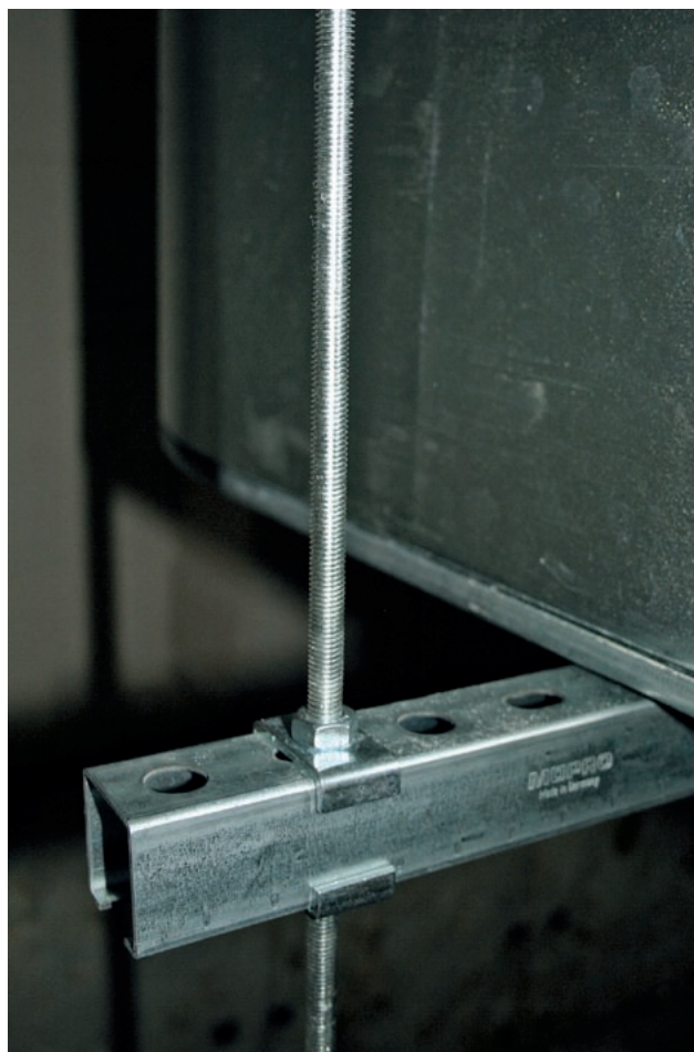
Obr. 12 Detail instalačního profilu pro vynesení čtyřhranného potrubí
