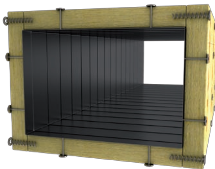
Obr. 36 Horní deska překrývá boční desky, které překrývají spodní desku
