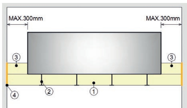
Obr. 43 Příčný řez svislým vzduchovodem s izolací z 1 strany
