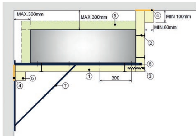
Obr. 78 Příčný řez potrubím s dvoustrannou izolací v místě požárně dělicí konstrukce
