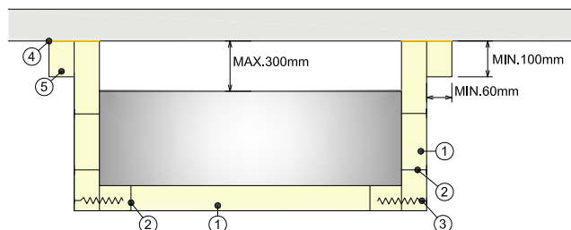
Obr. 45 Příčný řez svislým vzduchovodem s izolací na 3 stranách
