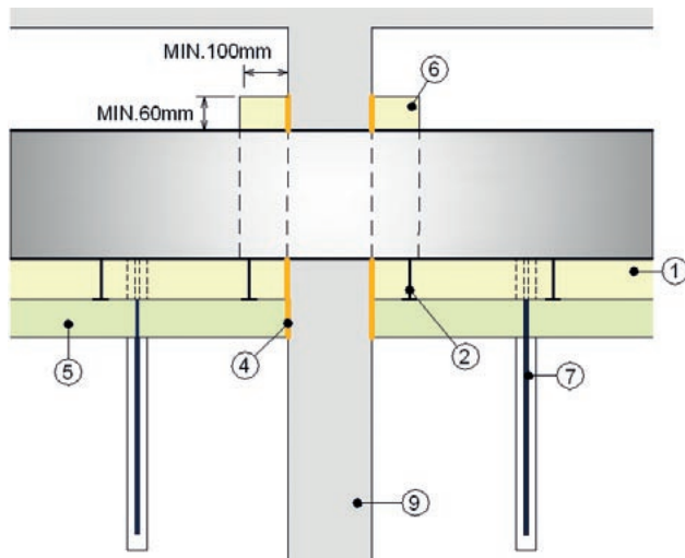
Obr. 48 Podélný řez vzduchovodem s izolací na 2 stranách procházející požárně dělicí konstrukcí
