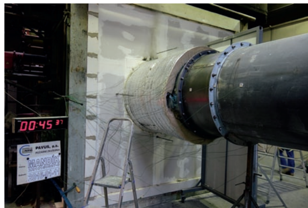
Obr. 82 Z materiálů Isover byl s předsazenými klapkami testován protipožární systém U Protect a to u výrobců MANDÍK, a.s. a Systemair a.s.
