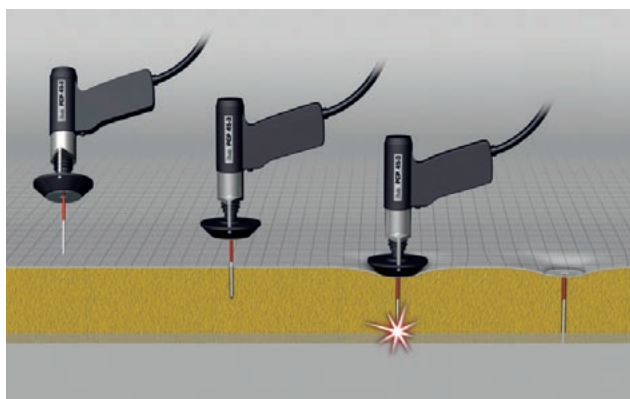
Obr. 15 Trn se vkládá podložkou do magnetické hlavičky pistole tak, aby bylo možno po propíchnutí izolace trnem provést jeho přivaření
