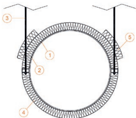
Obr. 29 Izolování potrubí s požární odolností EI 60 1 - VZT potrubí • 2 - dvoudílné objímky (např. MÚPRO) 3 - závitová tyč • 4 - lamelová rohož Orstech LSP PYRO tloušťky 50 mm • 5 - ochranný pás o rozměru 160 × 250 mm (nutný pouze u vodorovných potrubí pro požární odolnost EI 60)
