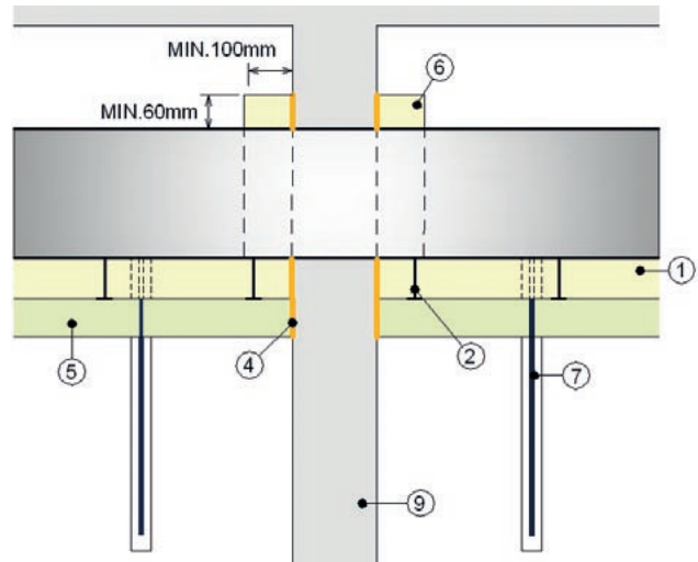
Obr. 79 Podélný řez potrubím s izolací na 2 stranách procházející požárně dělicí konstrukcí
