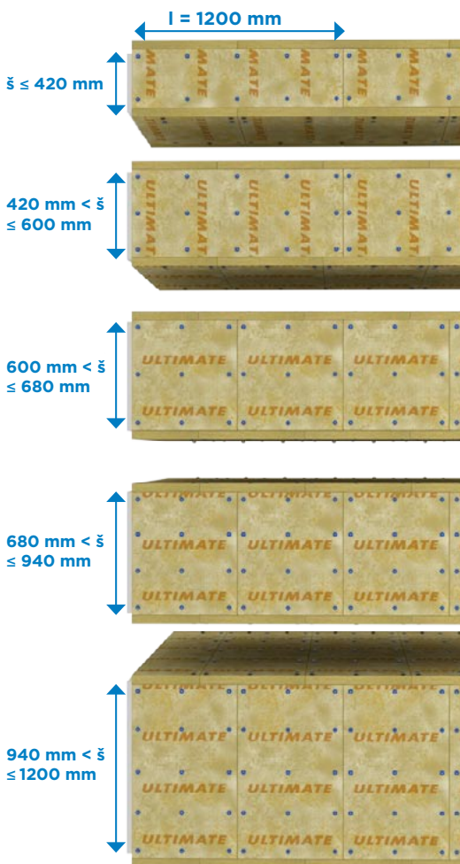
Obr. 67 Rozmístění trnů a vrutů u vodorovného potrubí
