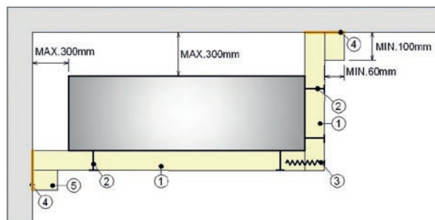
Obr. 75 Příčný řez potrubím s izolací na 2 stranách
