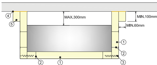
Obr. 76 Příčný řez svislým potrubím s izolací na 3 stranách
