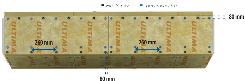
Obr. 37 Maximální vzdálenosti trnů a vrutů Fire Screw
