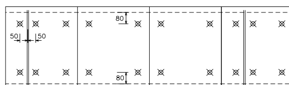
Obr. 17 Rozmístění trnů u čtyřhranného VZT potrubí
