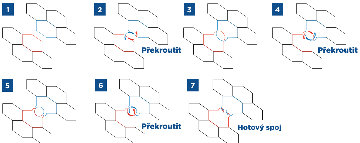
Obr. 55 Schematické znázornění principu spojení rohože na pletivu
