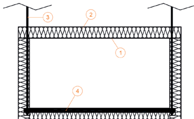
Obr. 24 Závitové tyče uvnitř izolace 1 - VZT potrubí 2 - desky Orstech 65 H tl. 40 (60) mm 3 - závitová tyč 4 - instalační profil (např. tvaru U 38/40 mm)
