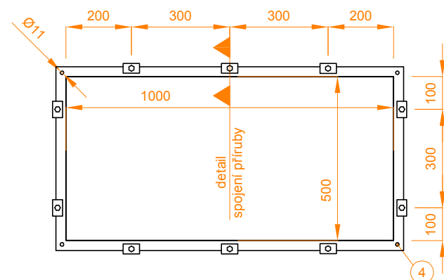
Obr. 10 Příruby zajištěné stahovacími svorkami
