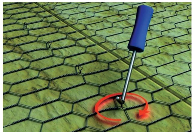
Obr. 54 Spojení rohoží překroucením přiléhajících okrajů pletiva do sebe po vzdálenosti cca 100 mm
