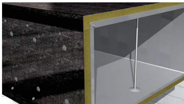
Obr. 58 Vyztužení segmentu potrubí uprostřed rozpětí
