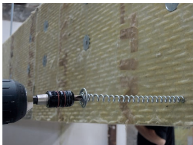
Obr. 65 Rohové styky desek jsou spojeny požárními vrtů Fire Screw
