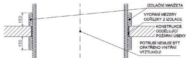
Obr. 25 Řez potrubím v místě prostupu požárně dělicí konstrukcí
