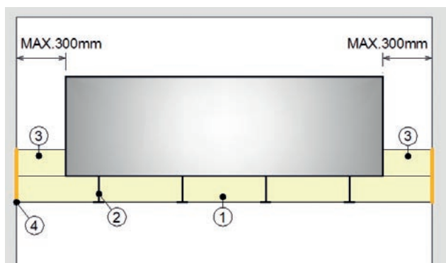
Obr. 74 Příčný řez svislým potrubím s izolací z 1 strany
