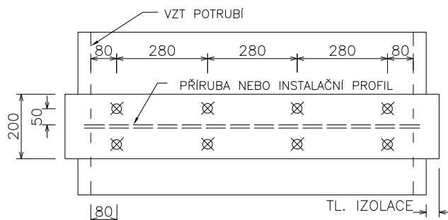
Obr. 20 Detail kotvení druhé vrstvy izolace, není-li zachováno krytí izolace nad přírubou nebo instalačním profilem min. tloušťky 20 mm
