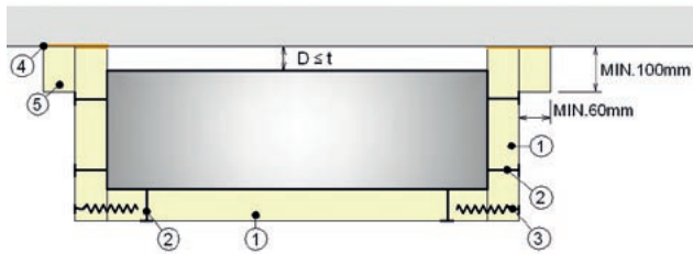
Obr. 77 Příčný řez vodorovným potrubím s izolací na 3 stranách
