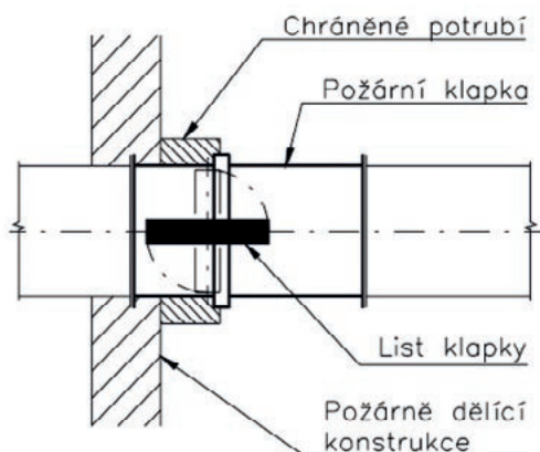
Obr. 81 Požární klapka zabudovaná mimo požárně dělicí konstrukci
