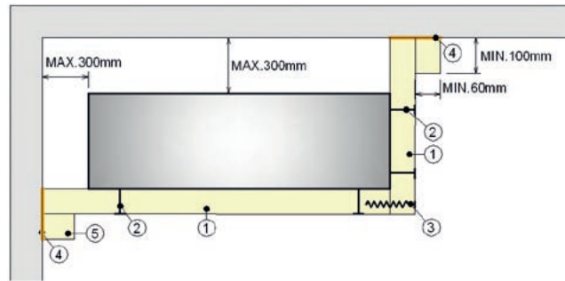
Obr. 44 Příčný řez vzduchovodem s izolací na 2 stranách
