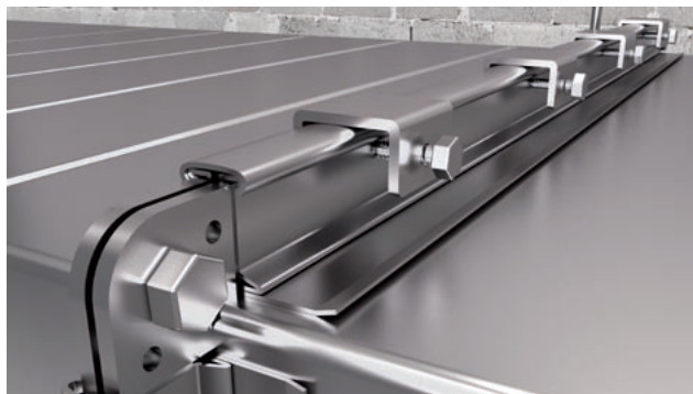
Obr. 60 Příruby zajištěné stahovacími svorkami
