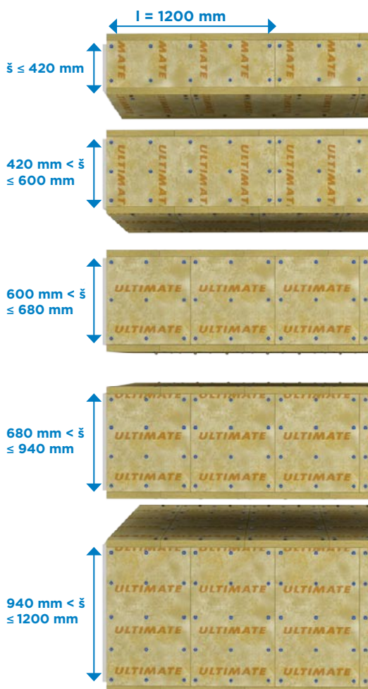
Obr. 38 Rozmístění trnů a vrutů u vodorovného potrubí
