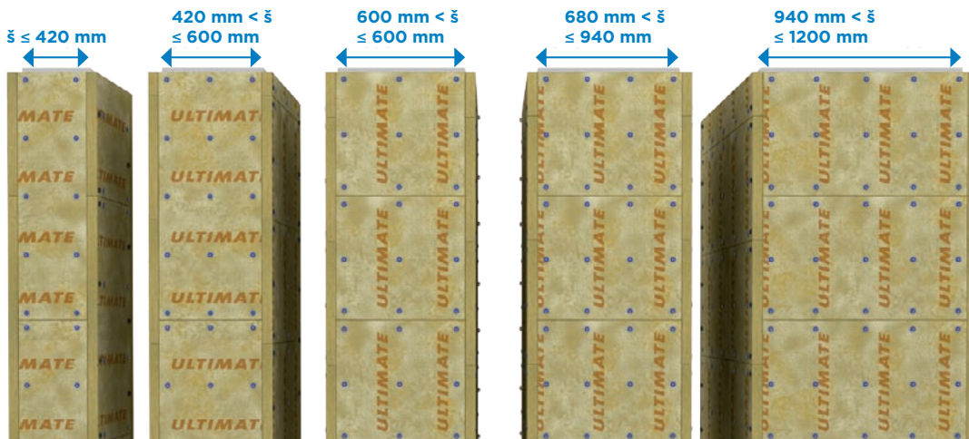
Obr. 68 Rozmístění trnů a vrutů u svislého potrubí
