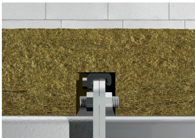
Obr. 19 Jednovrstvé kladení izolace v místě příruby - zachování min. tloušťky 20 mm nad přírubou
