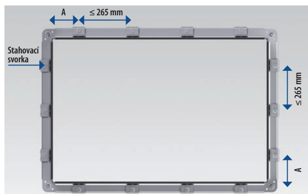
Obr. 34 Příruby zajištěné stahovacími svorkami
