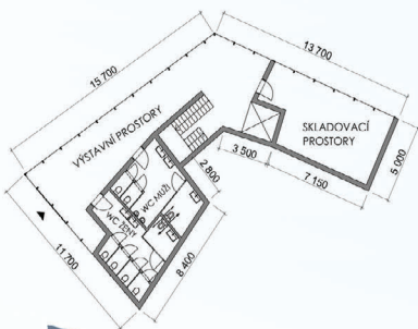
PŮDORYS SUTERÉNU
