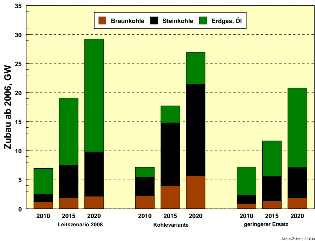
Abbildung 3.18: Bedarf an neuen fossilen Kraftwerken zwischen 2006 und 2020 im LEITSZENARIO 2008 und in zwei weiteren Varianten
