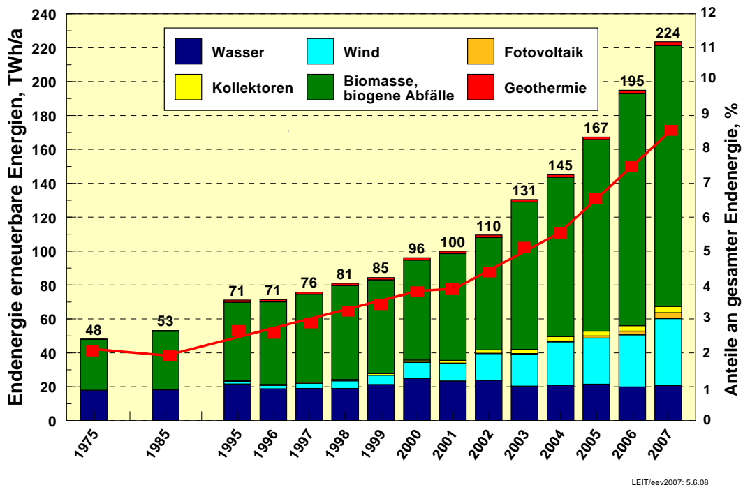
Abbildung 1.1: Gesamter Endenergiebeitrag erneuerbarer Energien nach Energiequellen 1975 – 2007 (Balken und linke Ordinate) sowie Anteile am gesamten Endenergieverbrauch (Kurve und rechte Ordinate). Quellen: Daten der AGEE-Stat. nach [BMU 2008a]; [BMWi 2008]; frühe Daten teilweise eigene Abschätzungen
