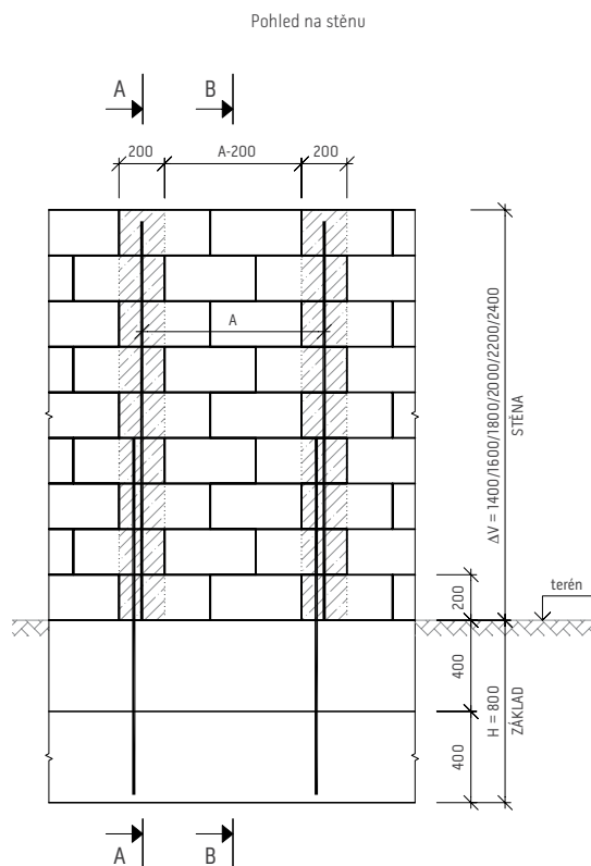
Schéma provedení stěny z tvárníc RONDE BLOCK – pohled, řez
