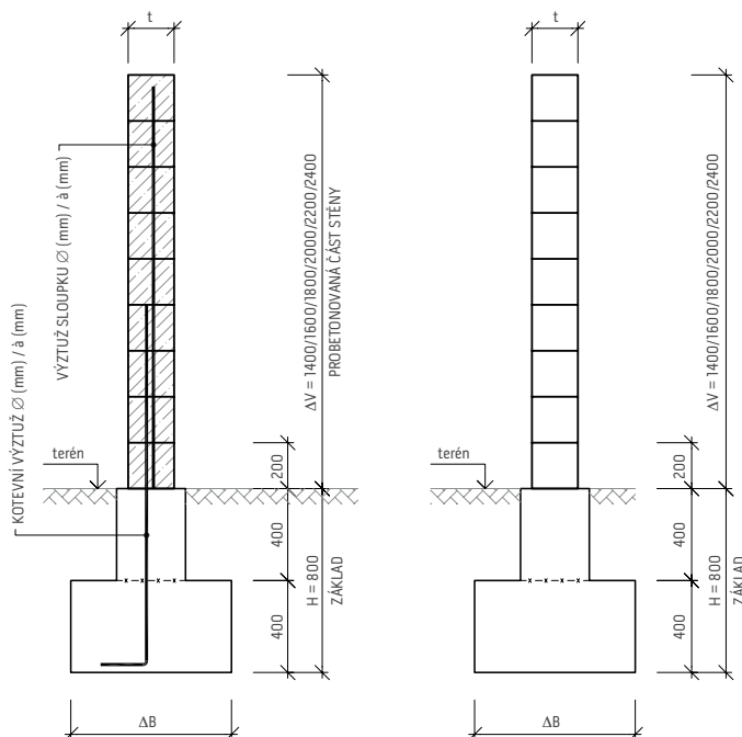
Řez A-A v místě probetonování
