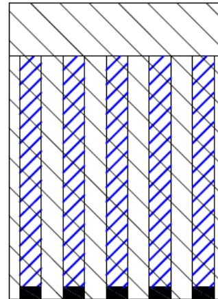
trubkový s válcovým absorberem
