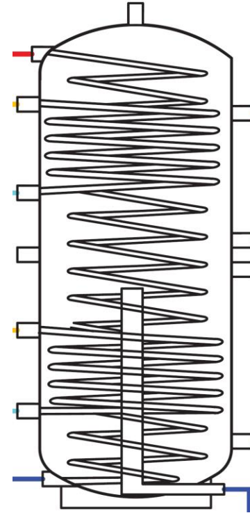
trubkový výměník
