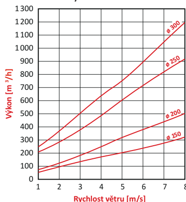
Graf výkonu:
